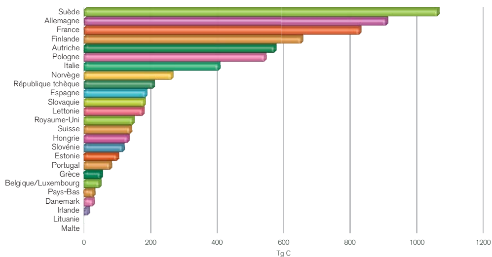
Carbone séquestré dans la biomasse ligneuse des forêts de l'UE
